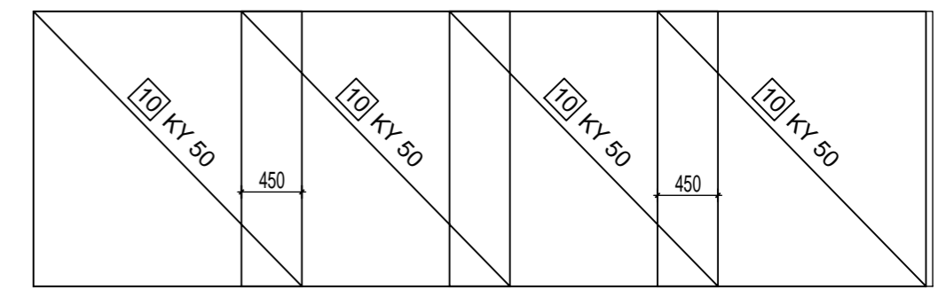
VÝSTUŽ PLECHODOSKY NA KÓTE +9,950
